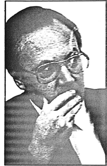
Eliseo Aja.
